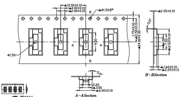
SB39SFTR
