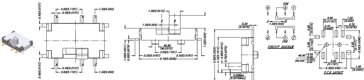
SB39DDTR 2P2T
